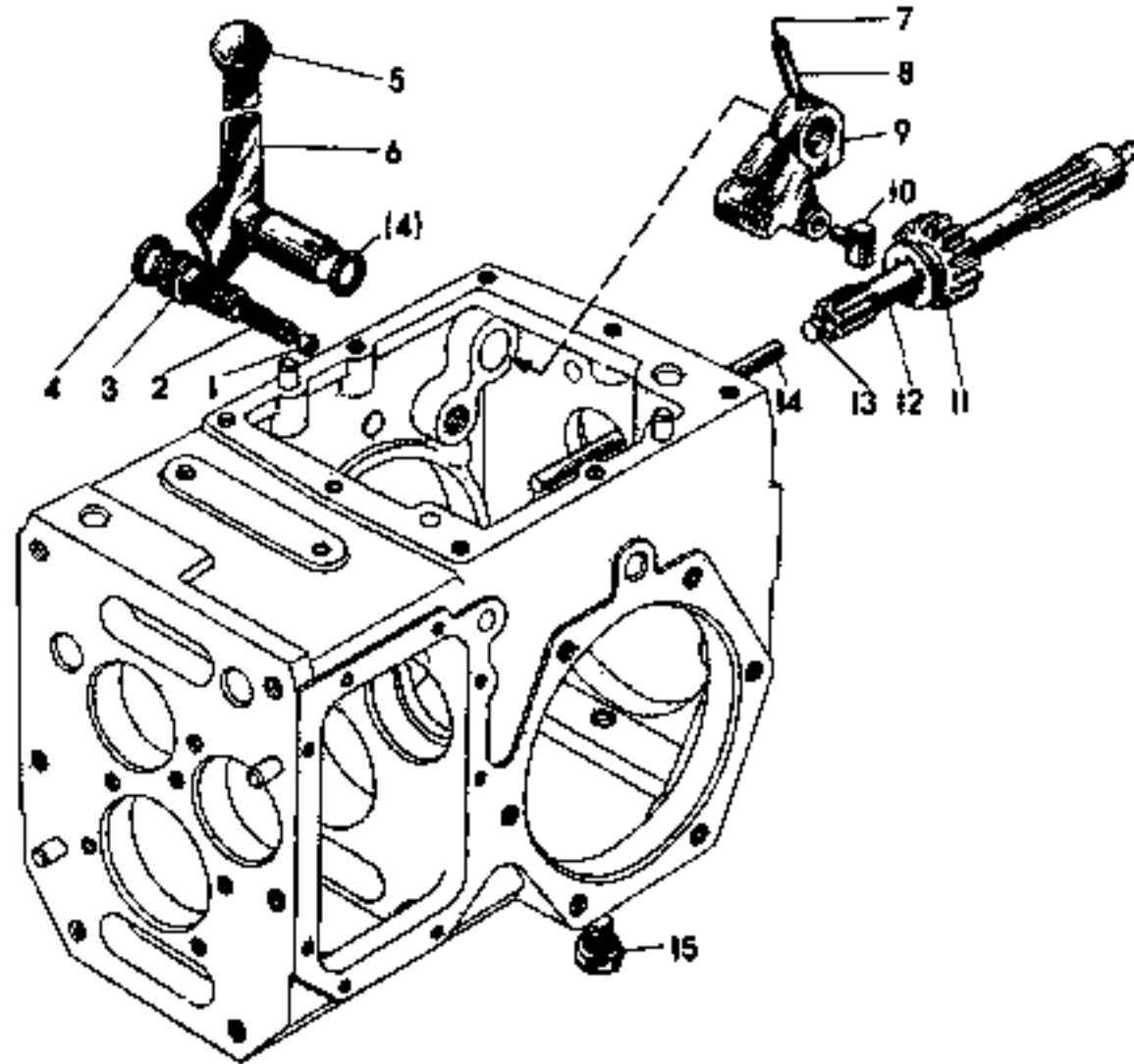
Рисунок 11 – Управление и привод БОМ
