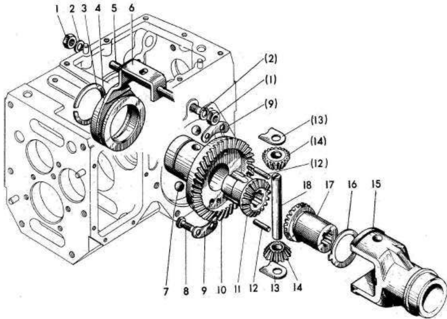
Рисунок 6 – Дифференциал
