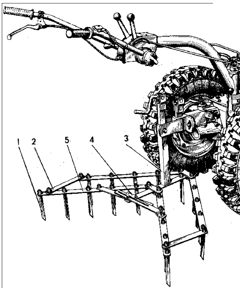
Рисунок 22 – Мотоблок в агрегате с бороней
