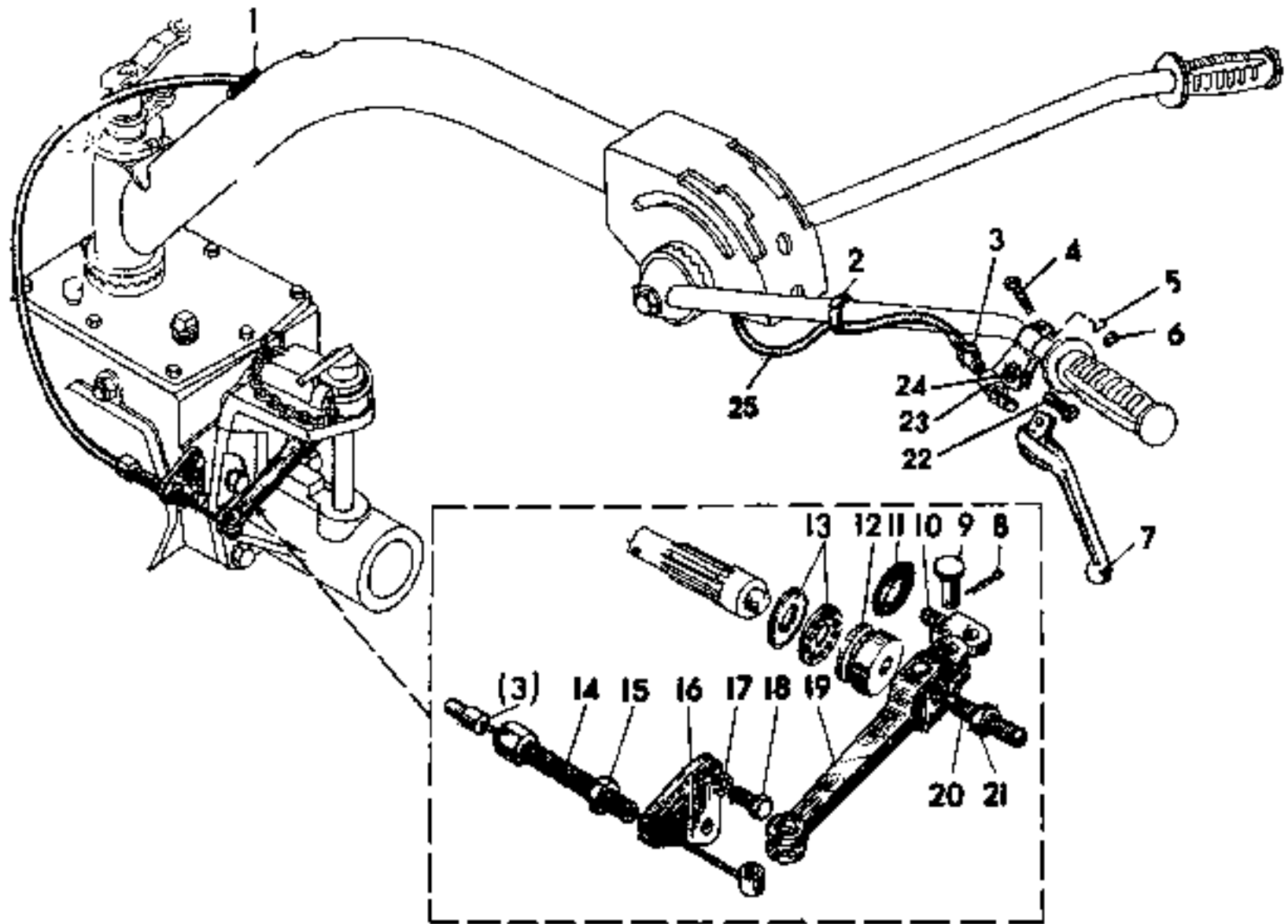
Рисунок 3 – Управление сцеплением
