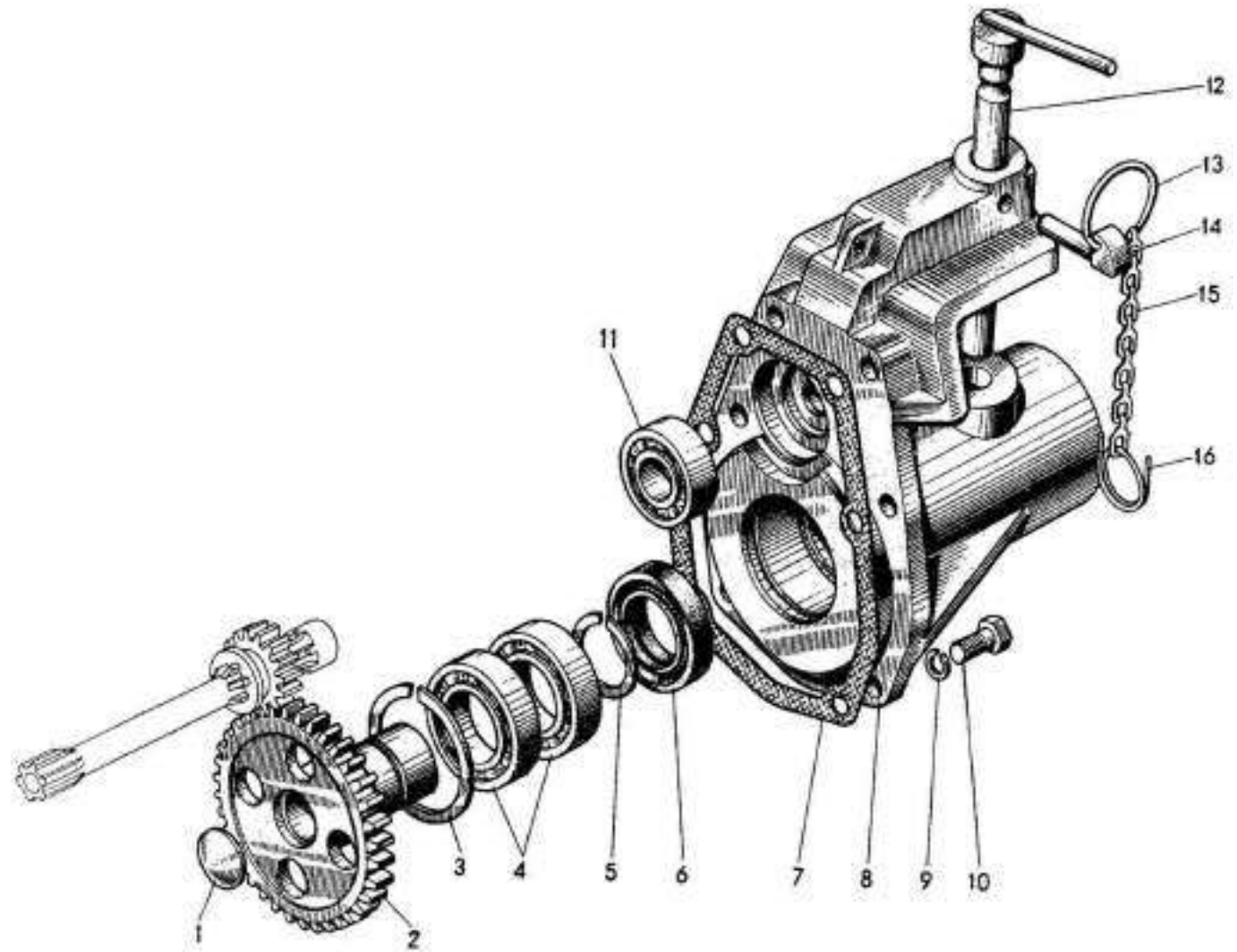
Рисунок 10 – Вал отбора мощности и прицепное устройство
