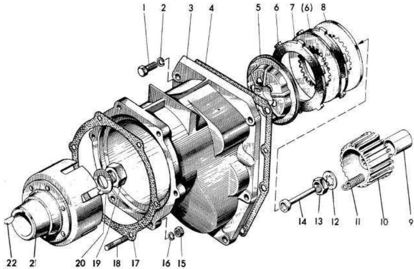
Рисунок 2 – Сцепление
